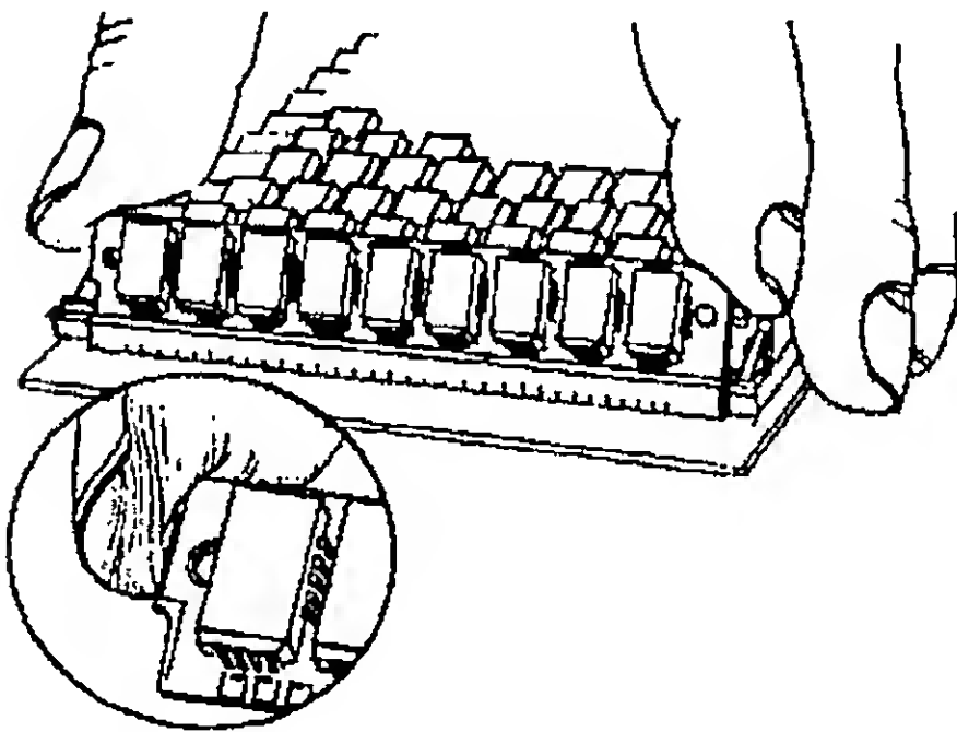
Figura 44 - encaixando um módulo de memória SIMM
